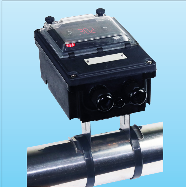
Ejemplo de montaje con soporte de montaje en la parte trasera en tubería horizontal
