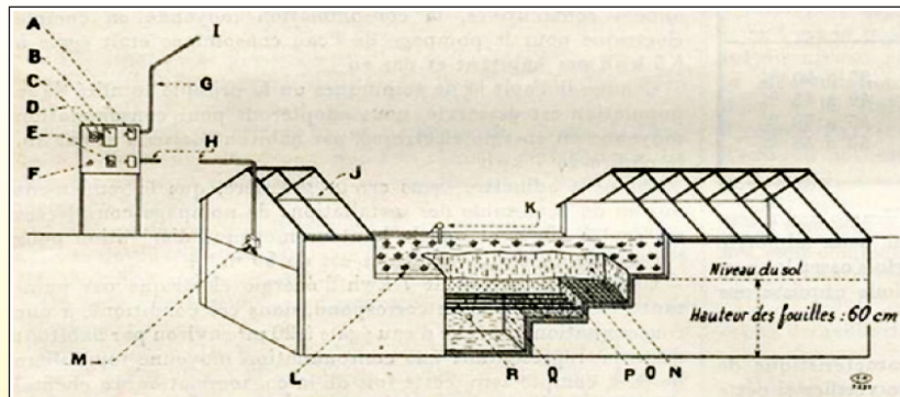
FIG. 1. — Coupe d'une bêche chauffée par câbles électriques.
