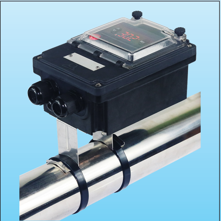
Ejemplo de montaje con soporte de montaje en la parte trasera en tubería vertical
